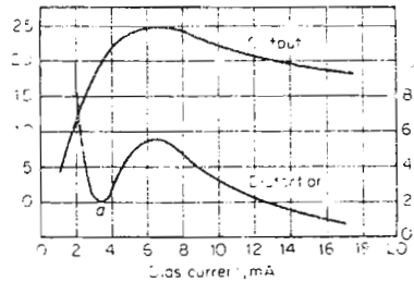
fig. 10-5. Livello del segnale in uscita e distorsione in funzione della corrente di polarizzazione.
