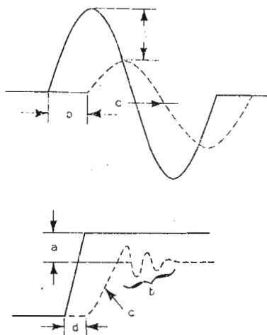
fig. 11.1 Distorsioni in un quadripolo lineare: - forma d'onda sinusoidale - forma d'onda a rampa
