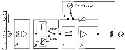
fig. 10-12. Riproduzione: Schema di principio
