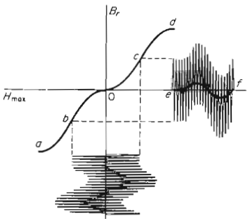
fig. 10-4. Registrazione lineare con addizione di portante di polarizzazione.
