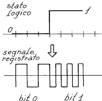
fig. 7.6 Modulazione bifase del codice binario
