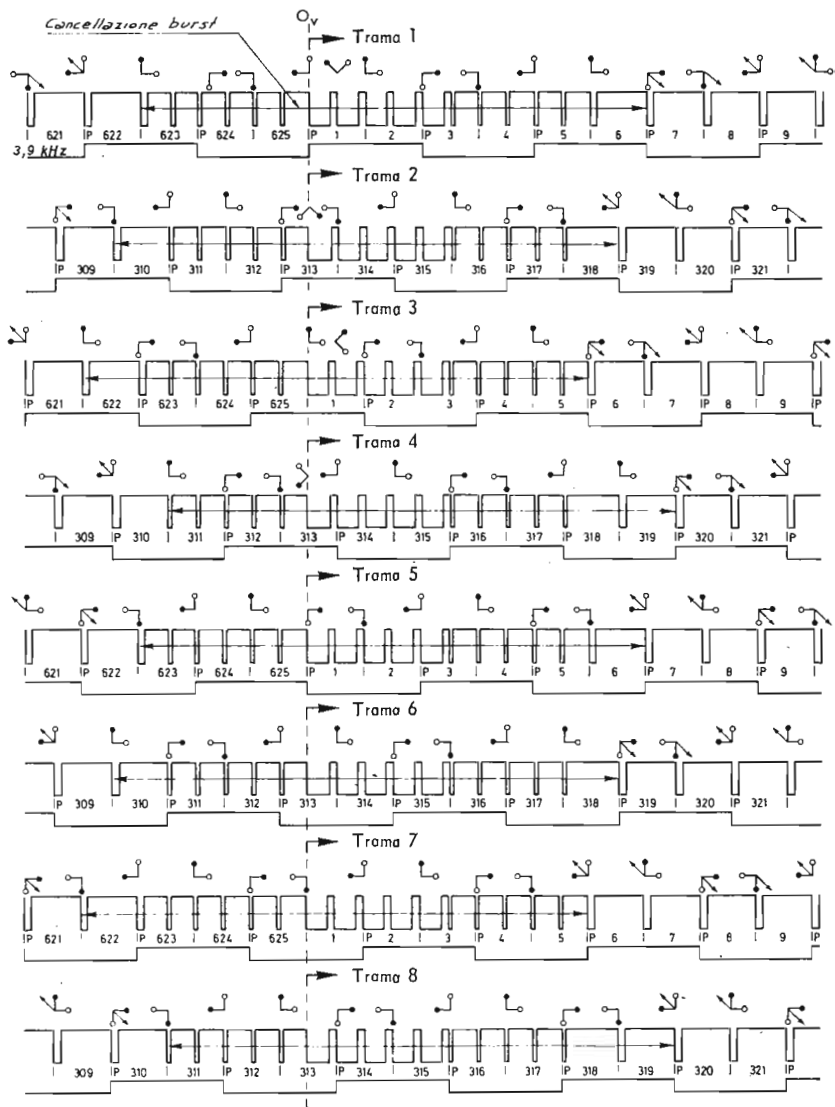
Rappresentazione vettoriale dei segnali Vettore E'v non invertito di segno a righe alternate • Vettore E'u — Burst P Riga sulla quale il vettore E'v non viene invertito di segno.
