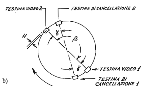
fig. 7.12 Registratore U-MATIC 3/4"
