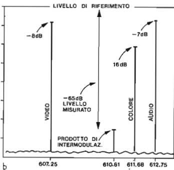
fig. 3.15 Misura della potenza e della intermodulazione
