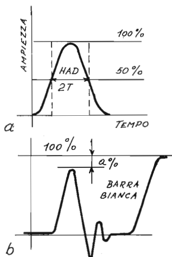
fig. 11.5 Impulso \text{sen}^2 2T (HAD = Half Amplitude Duration = Durata a mezza ampiezza): a - Forma indistorta paragonata con la corrispondente forma a trinangolo dell'impulso a rampa e con l'impulso rettangolare equinergetico ideale b - Forma distorta in ampiezza e in fase-frequenza
