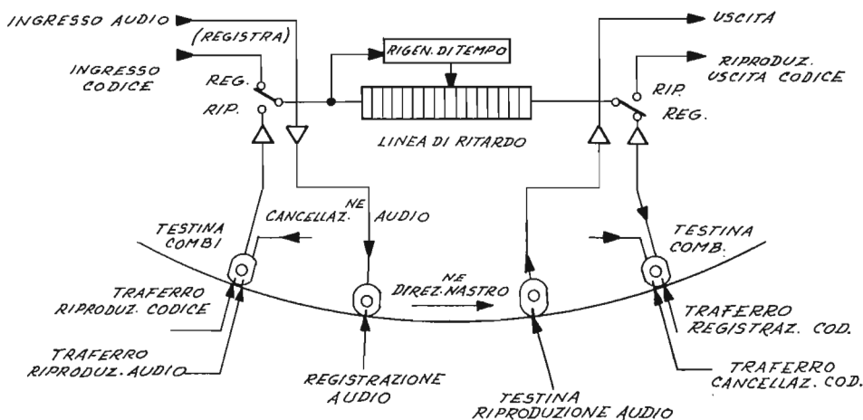
fig. 10-14. Schema di principio di registratore pilotato da codice SMPTE. (Studer).
