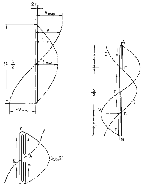
Fig. 2.3 Distribuzione di corrente e tensione lungo i dipoli: a) Dipolo \lambda/2 ; b) Dipolo ripiegato
