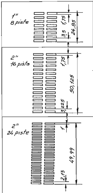
Fig. 10-10. Dimensioni delle tracce prodotte dai blocchi di testine multipista:
