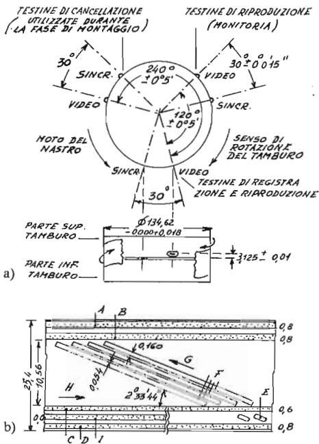
fig. 7.4 a: Configurazione del tamburo portatestine Standard C b: Posizioni normalizzate delle piste (quote in mm) A: pista audio 2; B: pista audio 1; C: pista di controllo; D: pista audio 3; E: pista di sincronismi; F: piste video; G: moto avanzamento testina; H: moto avanzamento nastro; I: pista audio 4 (in alternativa a E).
