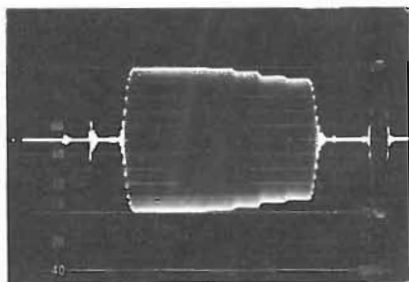
fig. 11.12 Segnale di cromaticità filtrato, affetto da distorsione di ampiezza
