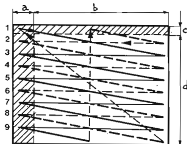
fig. 1.2 Quadro televisivo interlacciato: a: periodo di cancellazione di riga = 12 \mu\text{s} b: periodo attivo di riga = 52 \mu\text{s} c: periodo di cancellazione di quadro = 1,2 \text{ ms} d: periodo attivo di semiquadro = 20 \text{ ms}
