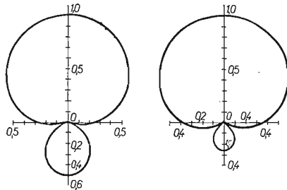
fig 9-5 Caratteristiche di microfoni super cardioide e ipercardioide
