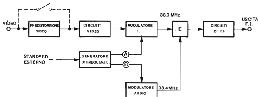
fig. 3.4 Schema a blocchi di modulatore a frequenza intermedia
