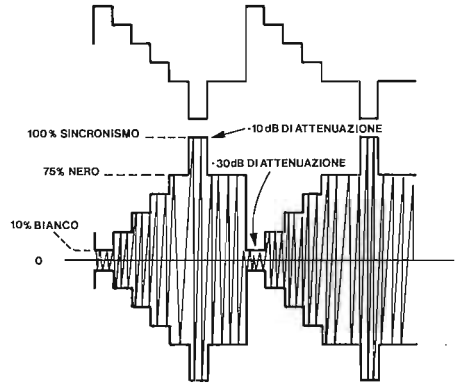
fig. 3.9 Involuppo di modulazione
