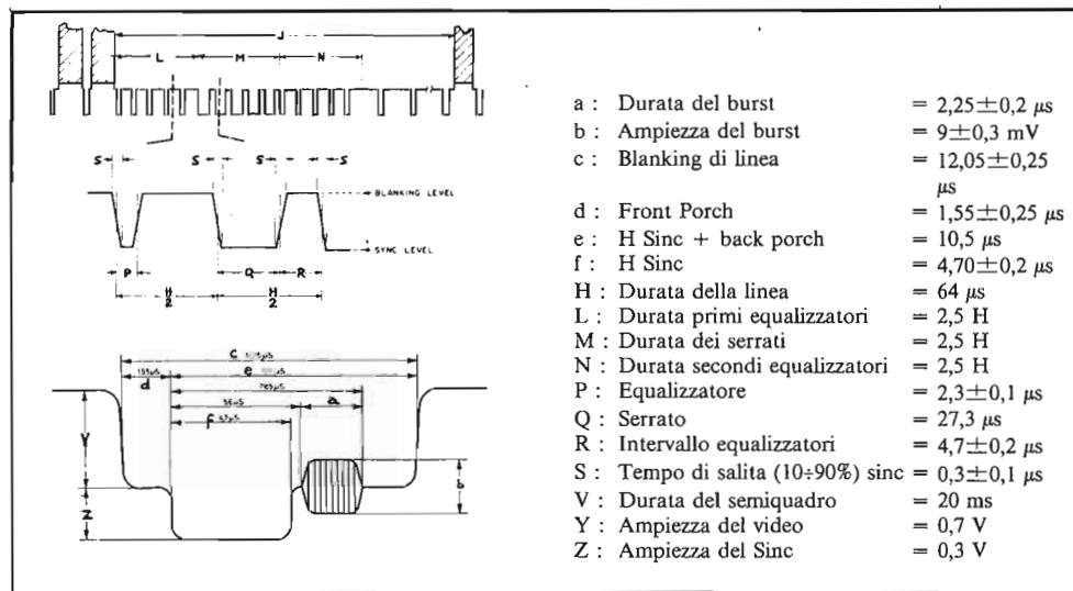
fig. 1.6 Durata e sequenze degli impulsi di sincronizzazione e degli impulsi colore PAL G/B:
