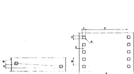
fig. 8-2. Dimensioni della pellicola 35 mm. Cinemascope a perforazioni CS.
