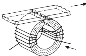
fig. 10-2. Testina di registrazione. Andamento delle linee di flusso.
