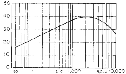
fig. 10-8. Caratteristica di risposta di frequenza per testina di lettura per la velocità di 7\frac{1}{2} al sec.
