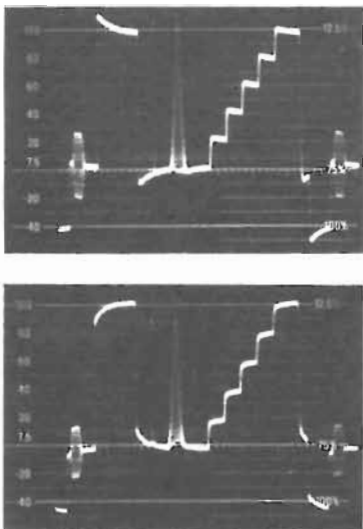
fig. 11.3 Distorsioni a frequenza di riga: a: overshoot (striscinamento di polarità opposta) b: streaking (striscinamento di uguale polarità)
