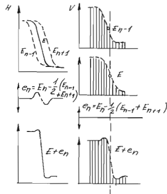
fig. 5.10 Curve di enfasi degli estrattori di contorni orizzontale e verticale
