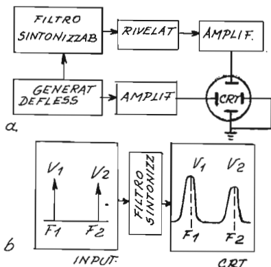
fig. 11.14 Analizzatore a filtro sintonizzato: a - Schema semplificato b - Forme d'onda
