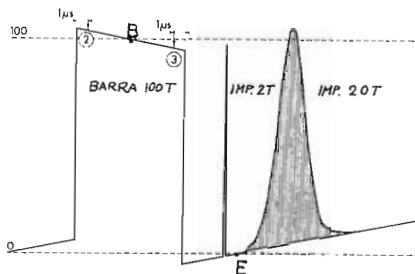
fig. 11.6 Misura dell'inclinazione della Barra di Luminanza
