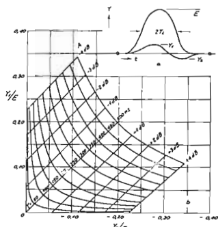
fig. 11.9 Grafico di calcolo K20T del ritardo di gruppo luminanza-crominanza
