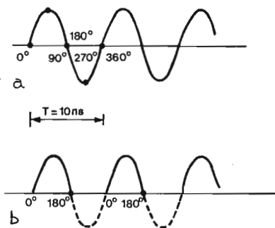
Fig. 3.30 a: funzionam. classe A (conduz. continua per 360°) b: funzionam. classe B (conduz. solo per 180°)
