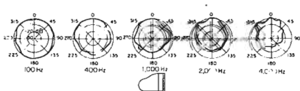
fig. 9-2 Direttività orizzontale di un pianoforte a coda
