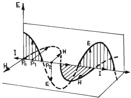
Fig. 2.2 E = Vettore elettrico H = Vettore magnetico I = Vettore induzione
