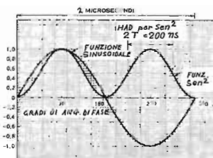
fig. 11.4 Comparazione tra le forme d'onda di \text{sen } \theta e \text{sen}^2 \theta
